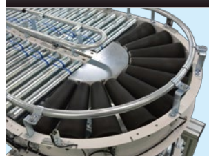
■ 業界最小 内Rのカーブコンベヤ
